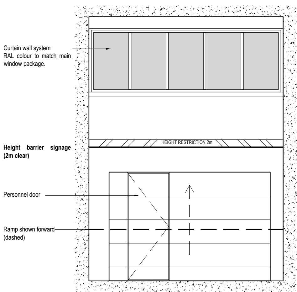
3 Elevation 1:50
